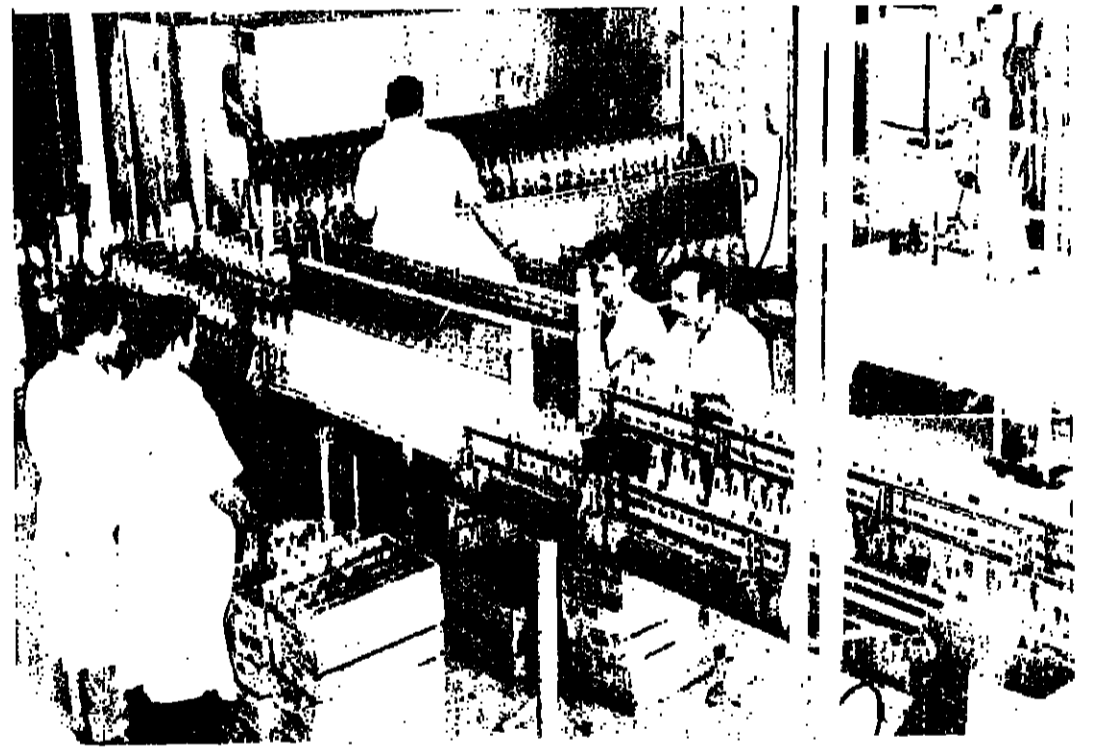
العمال الذين مهمتهم مراقبة الزجاجات وهي تسمى بطريقة أوتوماتيكية على شبكة الإنتاج ..
